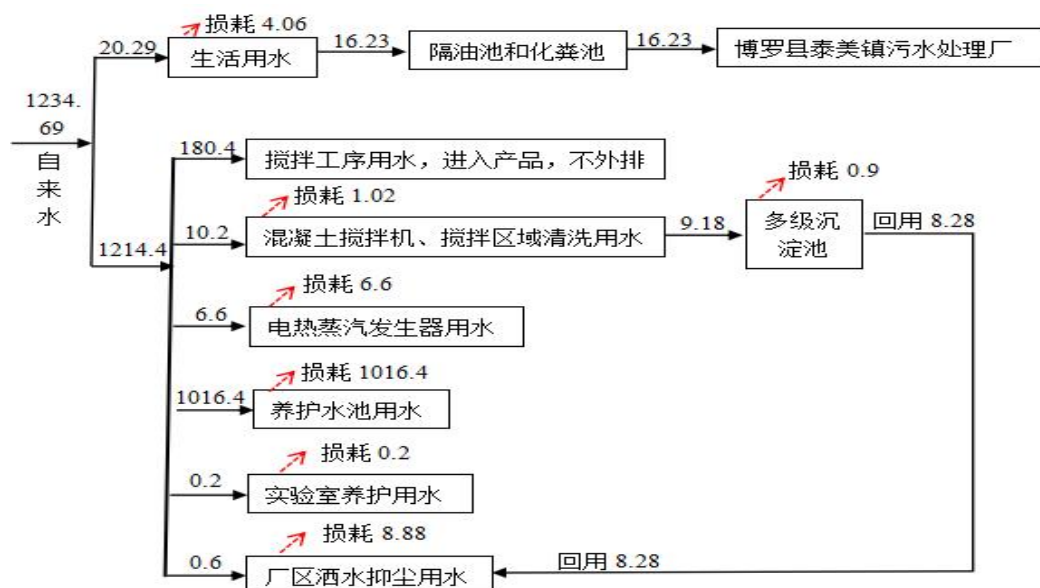
图 2-1 项目水平衡分析图 (单位 m 3 /d)
