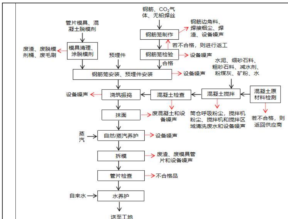
图 2-3 钢筋混凝土管片生产工艺流程图
