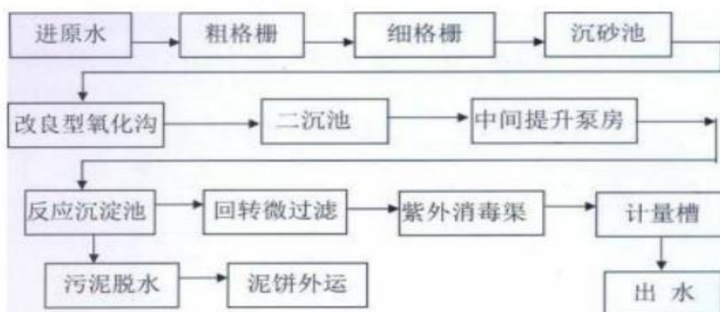
图 4-1 博罗县泰美镇污水处理厂废水处理工艺流程图
